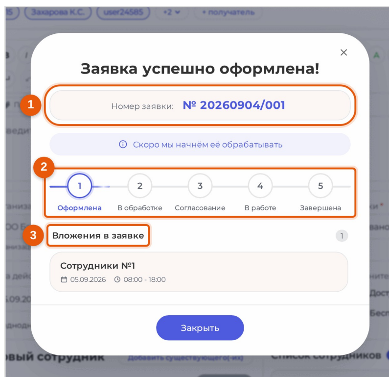
Рисунок 4.15 — Заявка отправлена
