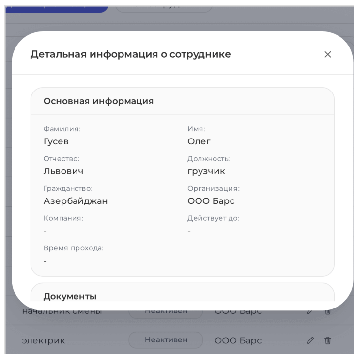
Рисунок 7.6 — Карточка сотрудника
